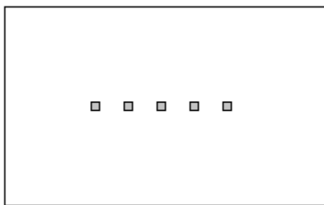
Bilde 7 – opphavstall som tallmengde
