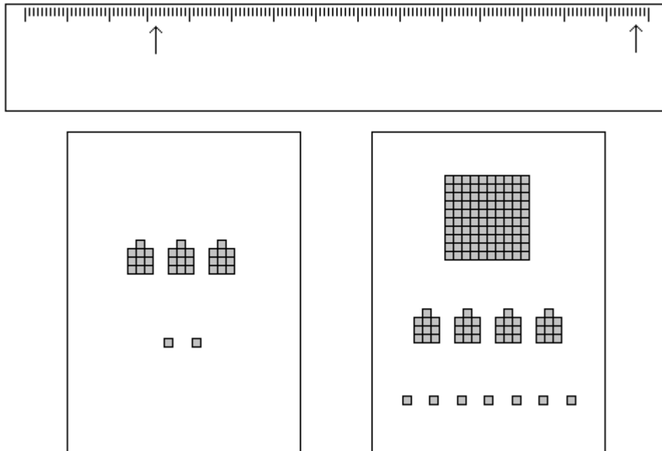
Bilde 7 – Linjal og tallmengder
